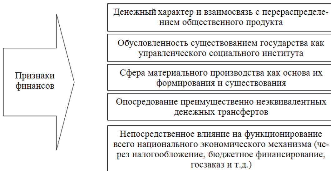
Рис. 1.1. Признаки финансов
