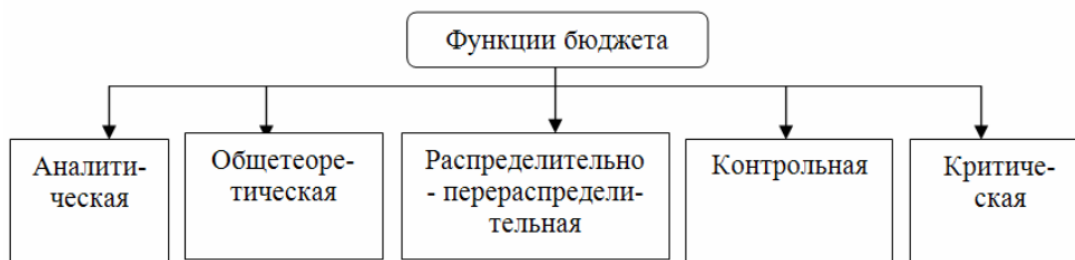
Рис. 1.14. Функции бюджета
